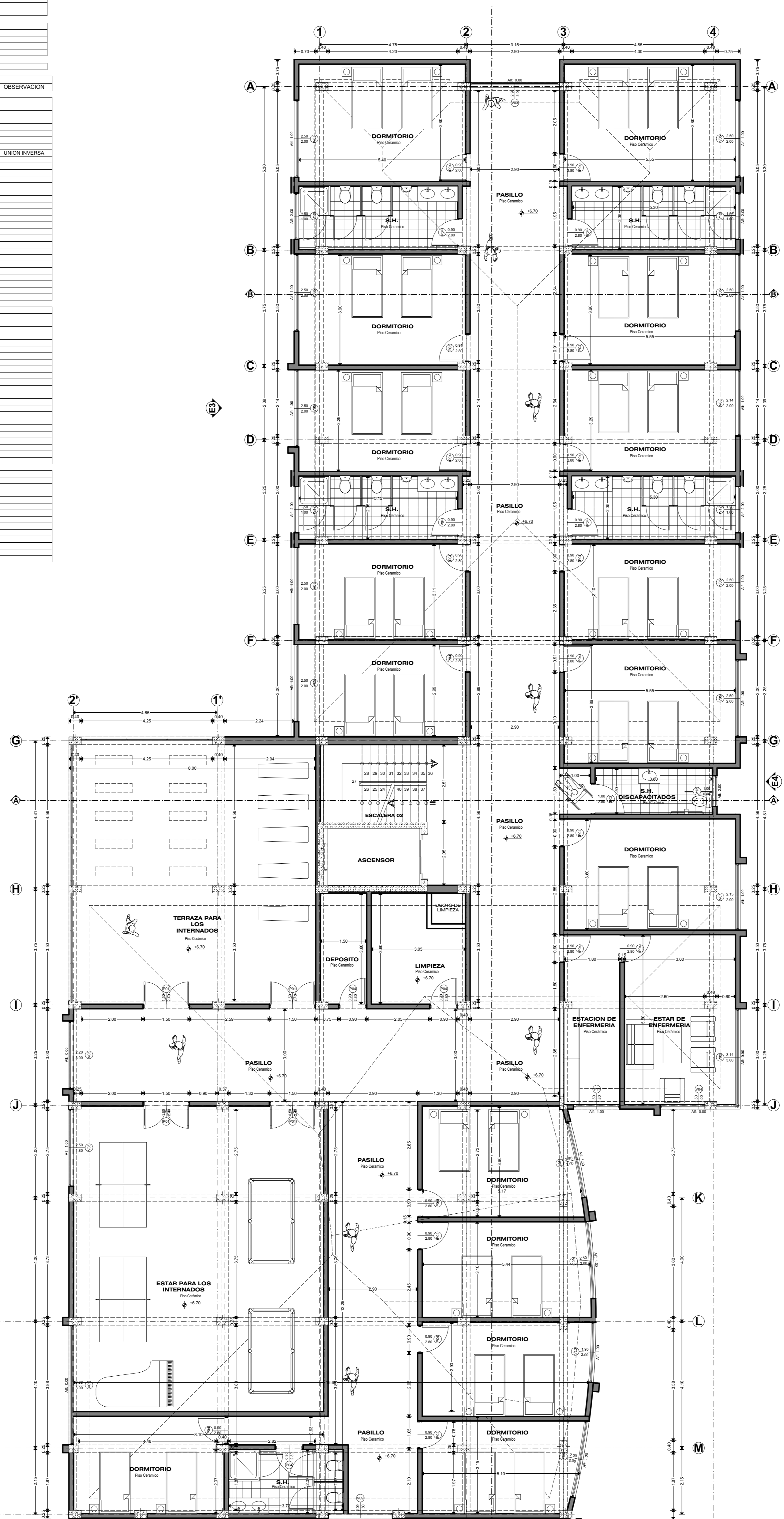
TERCER NIVEL ZONA DE INTERNAMIENTO Esc: 1:75
