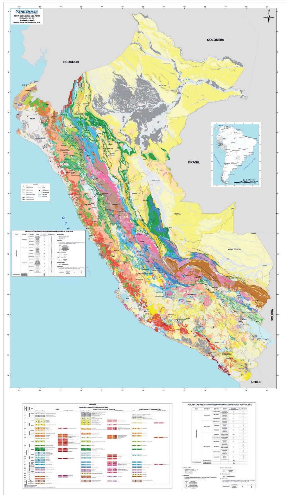
Figura 3. Mapa Geológico
